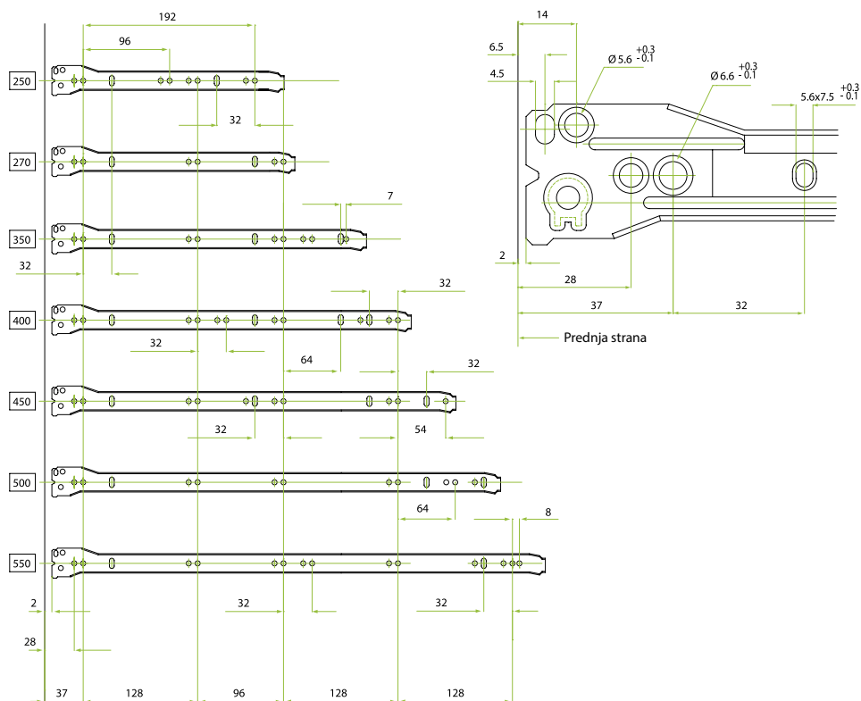
Klizači za Metalbox
