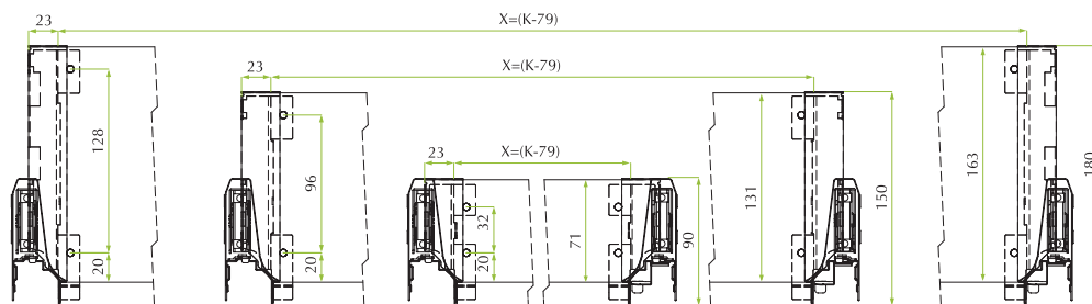
Pogled od pozadi
