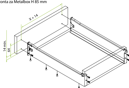
Montaža fronta za Metalbox H 85 mm
