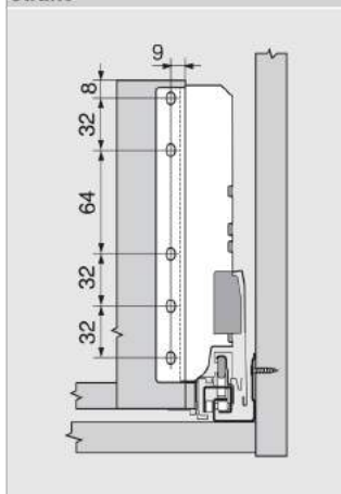
Dimenzije za ugradnju zadnje strane
