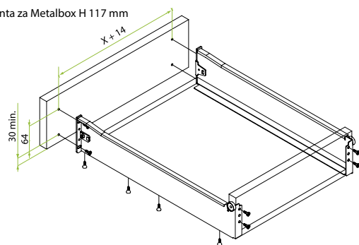
Montaža fronta za Metalbox H 117 mm
