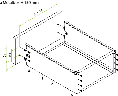
Montaža fronta za Metalbox H 150 mm
