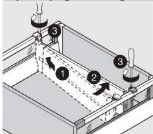
Poprečna pregrada sa mogućnošću pregrađivanja
