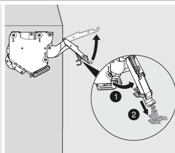
Polugu pažljivo otvoriti
