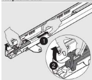
Uklanjanje osigurača za transport
