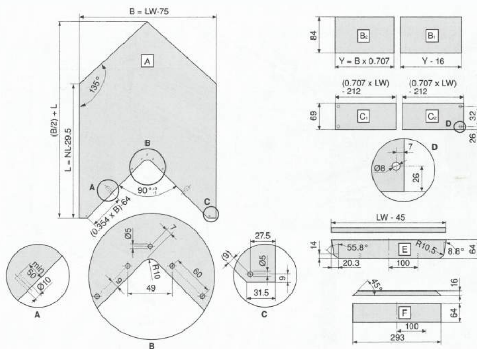
Dimenzije za krojenje za 16mm ploča od iverice
