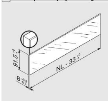
Dimenzije za krojenje uložnog elementa
