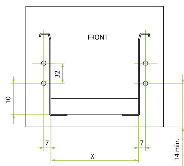
Šablon za bušenje
