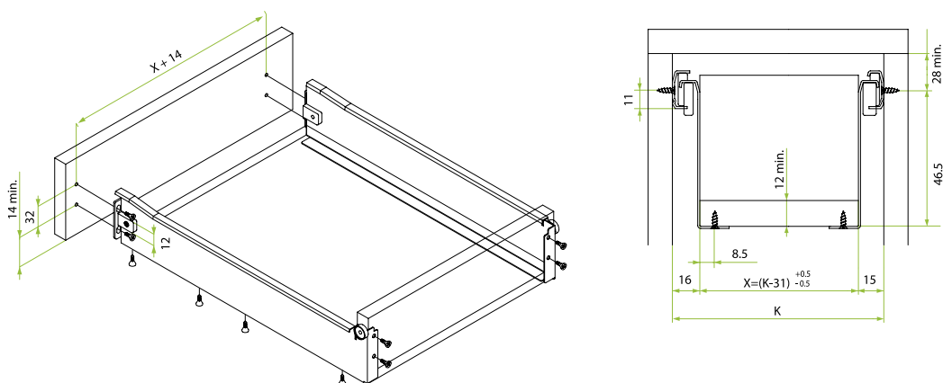
Montaža fronta za metalbox H - 53 mm
