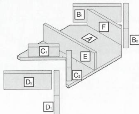
Dimenzije za krojenje za 16mm ploča od iverice
