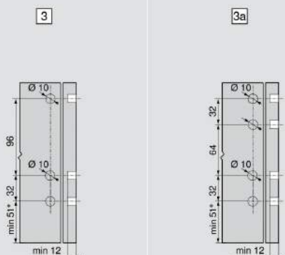
Dimenzije za bušenje otvora frontova za EXPANDO
