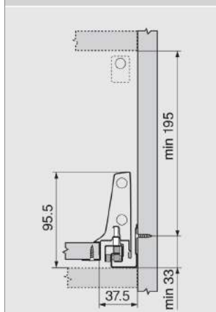
Pozicija za zavrtnje za šine korpusa
