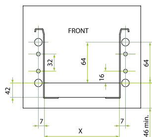
Šablon za bušenje
