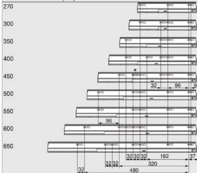
Dimenzije za krojenje uložnog elementa
